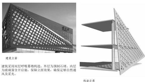
图 1: 双层遮阳通风式呼吸幕墙
