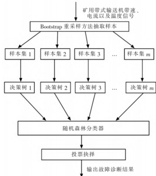
图7 煤矿带式输送机故障诊断模型图
