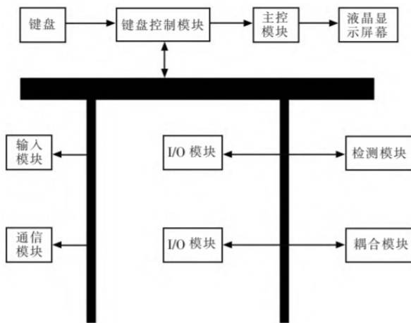
图4 工控操作台架构图
