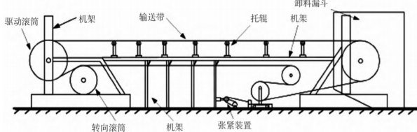
图1 煤矿带式输送机结构图
